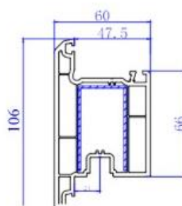
60 Outward Door Sash 411300
