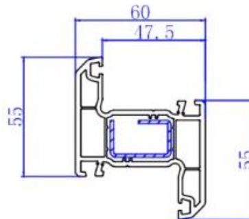
60 Outward Door Sash 411300
