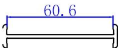
60 Bar 420200
