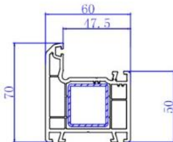
60 Door Frame 410500
