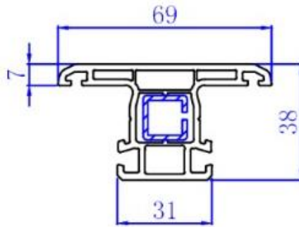
Sliding Door Sash 411900
