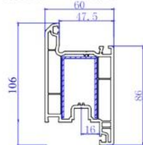
60 Inward Door Sash 410600
